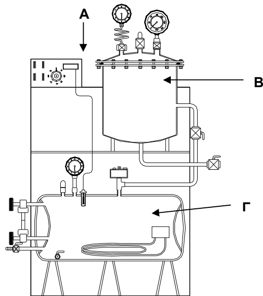
Εικόνα 4: Συσκευή υδροθερμικού χειρισμού που χρησιμοποιείται για την ανάκτηση ξυλοτεμαχιδίων από παλιές ξυλοπλάκες. Α: Πίνακας Ελέγχου, Β: Αντιδραστήρας, Γ: Μονάδα παραγωγής ατμού (Lykidis 2004).
