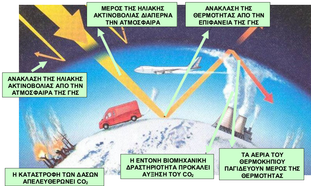
Εικόνα 1: Το φαινόμενο του θερμοκηπίου (Pearse 2002).
