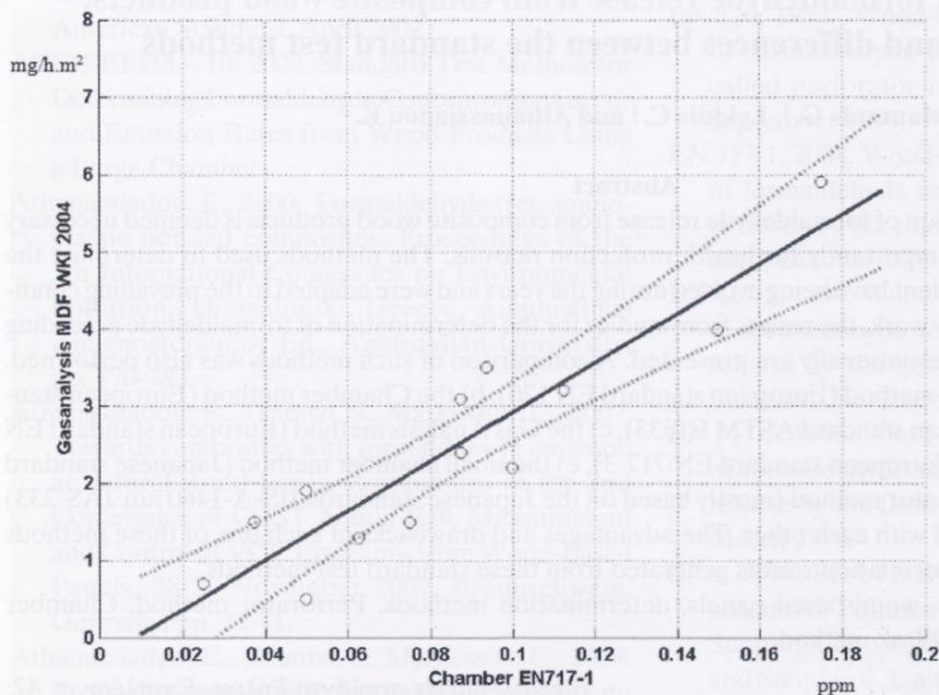
Σχήμα 5. Καμπύλη συσχέτισης μεταξύ της μεθόδου αεριοανάλυσης και της μεθόδου θαλάμου για MDF (πηγή: Schwab et al. 2007, Ινστιτούτο WKI Γερμανίας).
