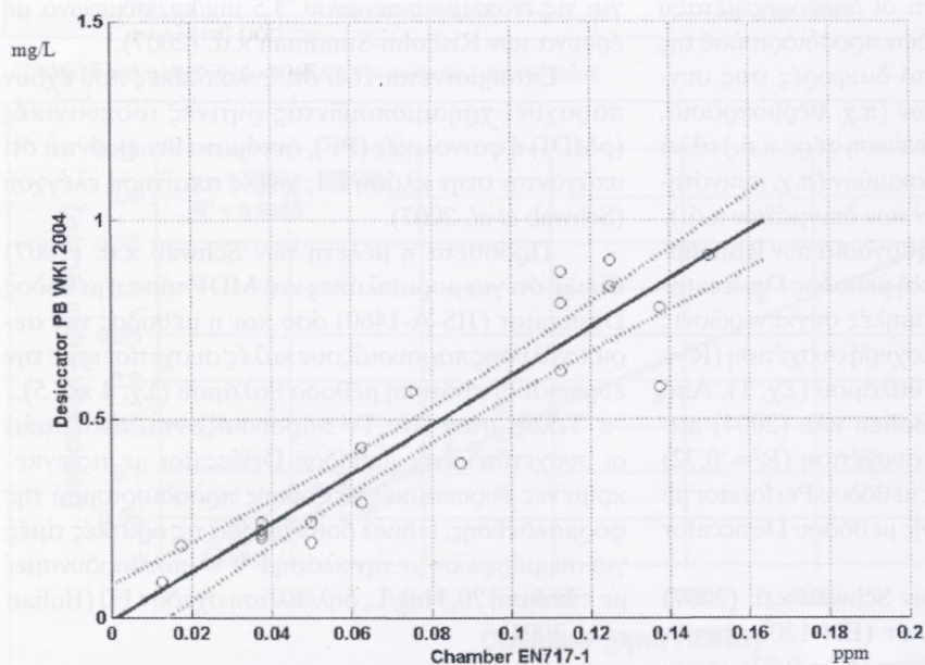
Σχήμα 4. Καμπύλη συσχέτισης μεταξύ της μεθόδου Desiccator και της μεθόδου θαλάμου για μοριοπλάκες (πηγή: Schwab et al. 2007, Ινστιτούτο WKI Γερμανίας).
